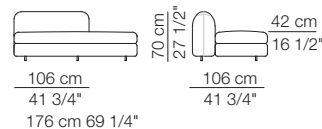
Elemento isola senza braccioli Isle unit without armrests
