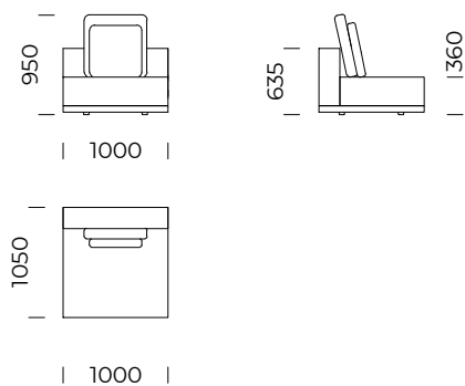
Siedzisko centralne A1 / Central seat A1
